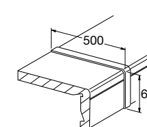
Profily připojení okenního parapetu
