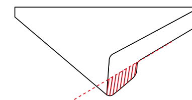
Frézování přední hrany do ztracena****
